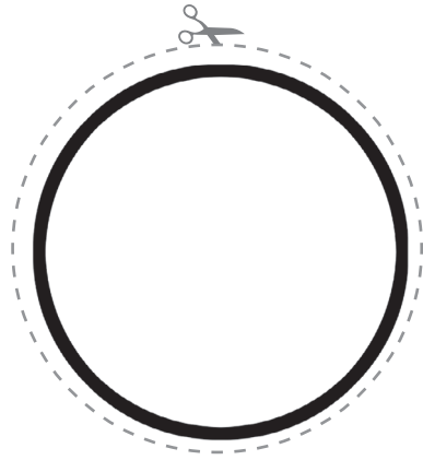
Jupiter
