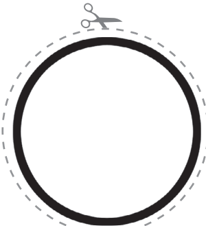
Venus
