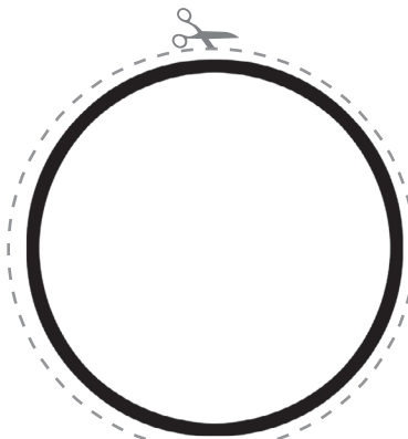
Uranus
